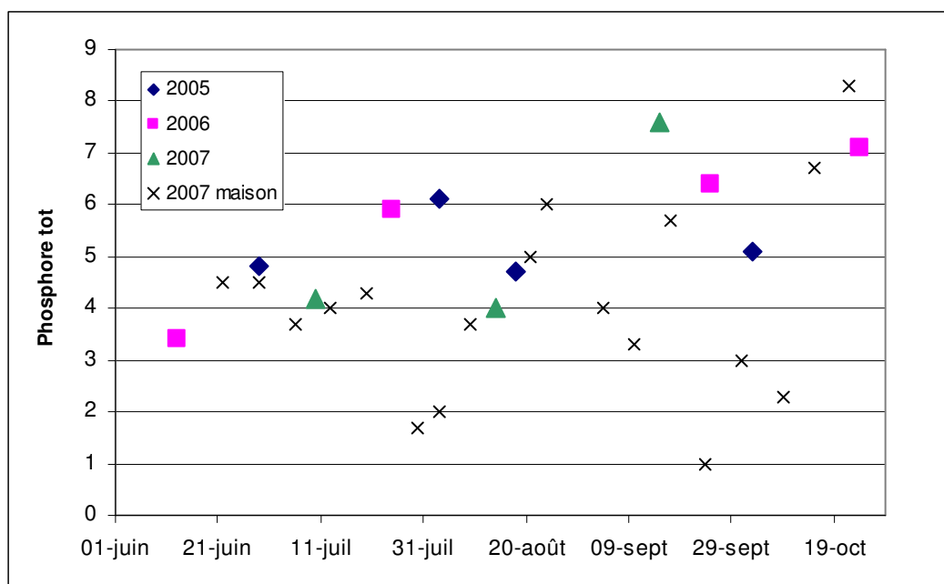
Figure 3.1 Phosphore total à l'effluent (mg / L)
