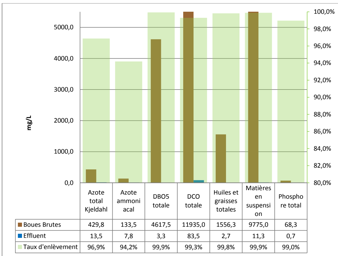
Figure 4 - Taux d'enlèvement 2015, de la boue brute à l'effluent traité, données moyennes
