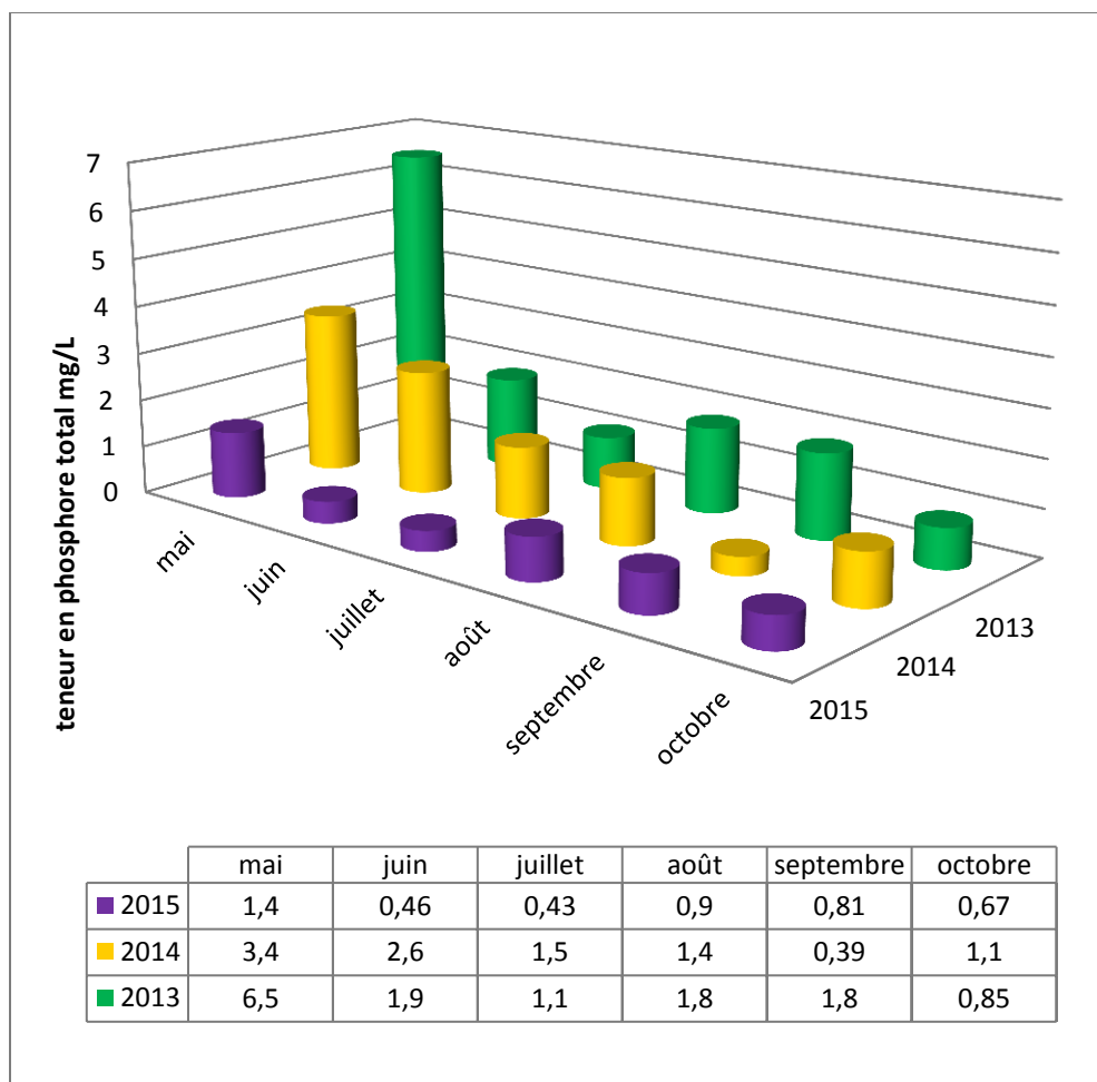
Figure 2 - Concentration en phosphore total (mg/L) de l'effluent
