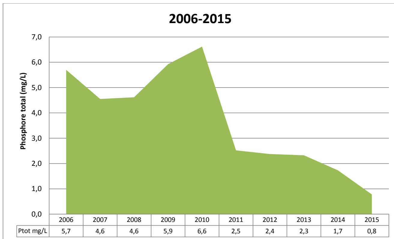
Figure 3 - Évolution de la concentration du phosphore de l'effluent
