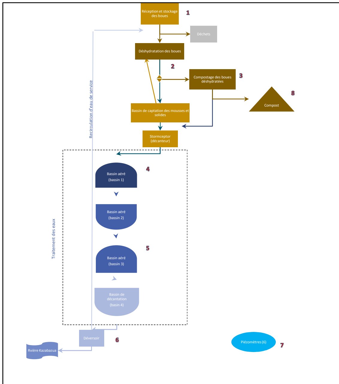
Figure 5 - Schéma en blocs des points d'échantillonnage
