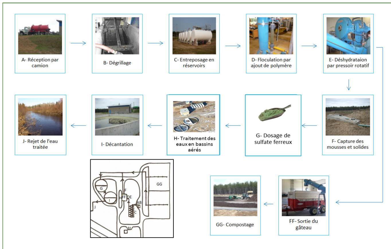
Figure 1 - Schéma de procédé illustré
