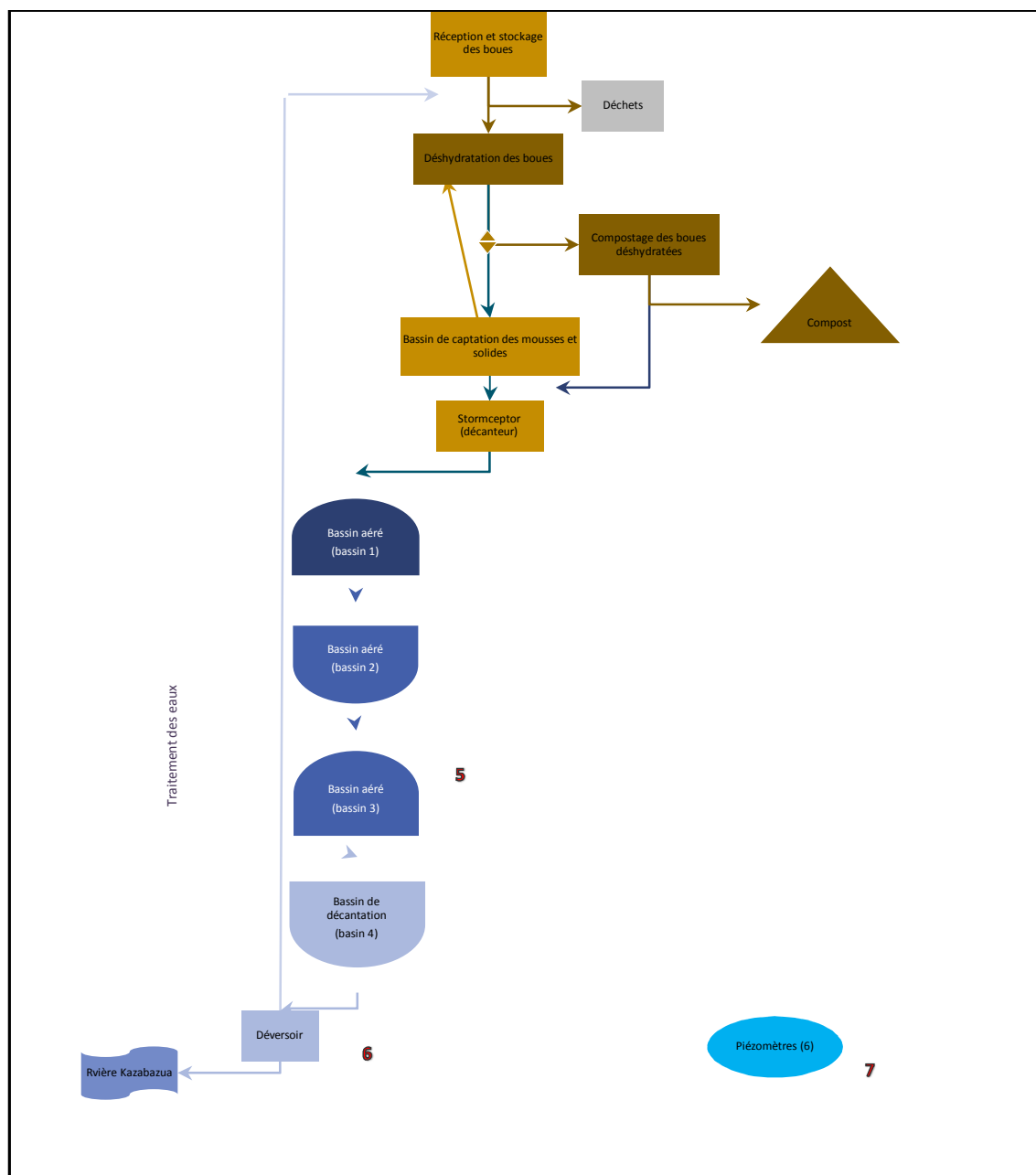
Figure 5 - Schéma fonctionnel des points d'échantillonnage
