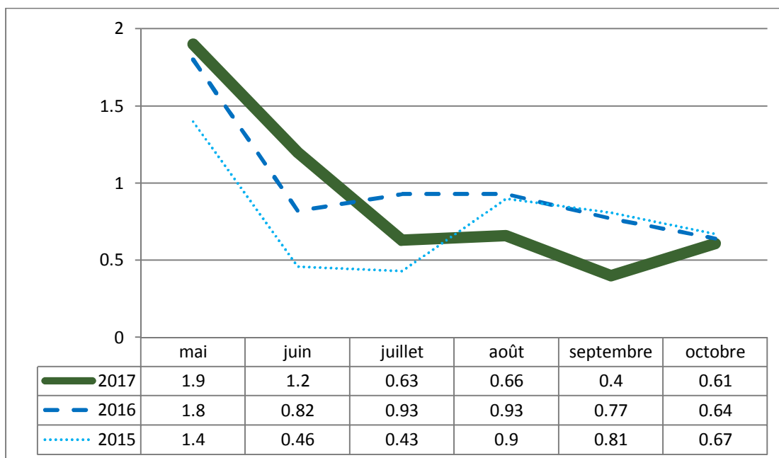
Figure 4 - Concentration de l'effluent en phosphore total
