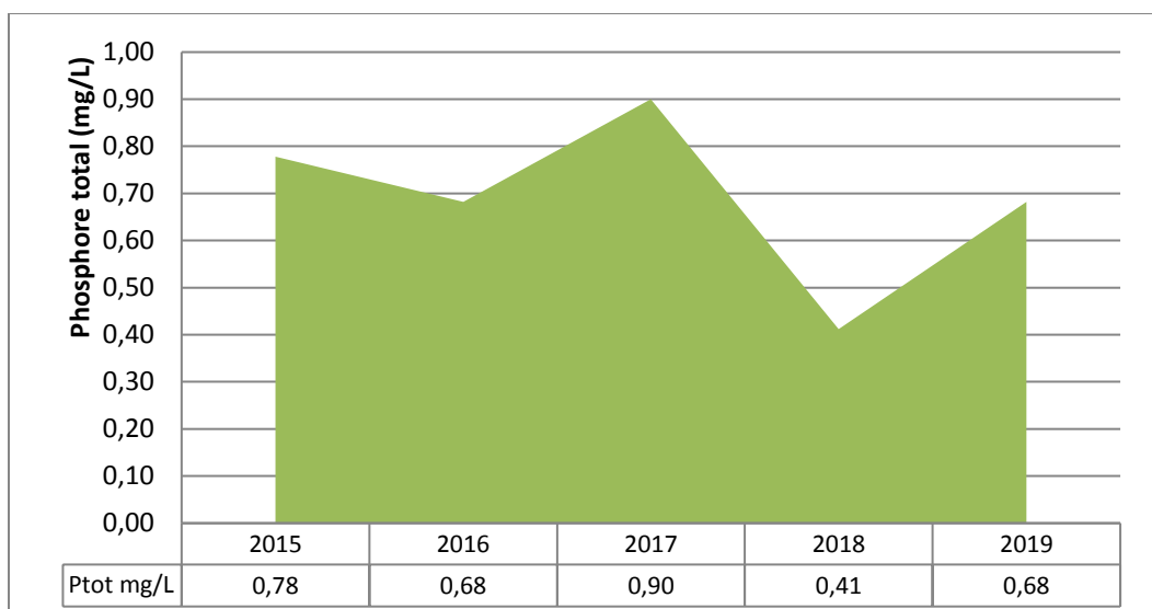
Figure 4 - Concentration moyenne annuelle en phosphore total à l'effluent (2015 à 2019)
