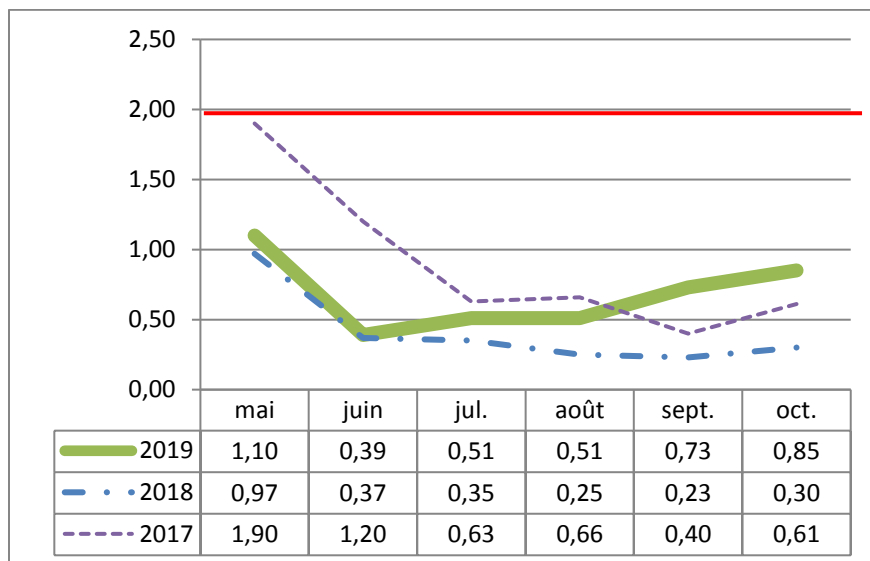
Figure 3- Concentration en phosphore total à l'effluent par mois (2017 à 2019)
