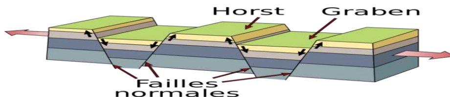
Figure 6.25 : Coupe transversale d'un ensemble de horsts et de grabens
